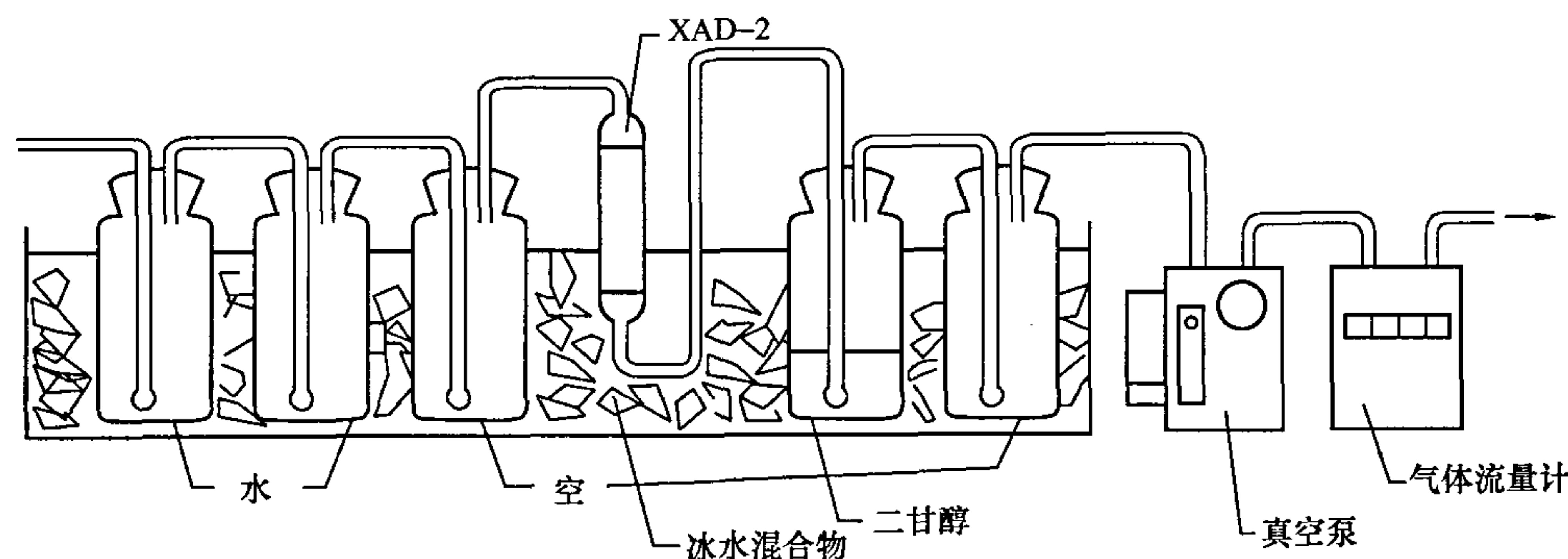
图 B.2 废气采样装置 I
