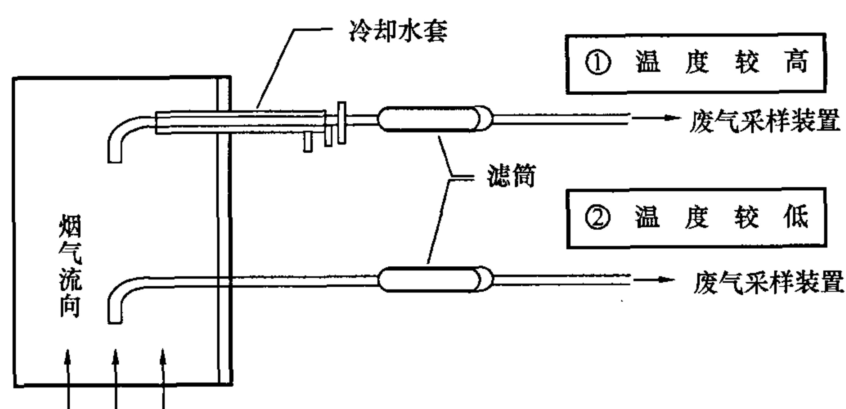
图 B.1 采样管和滤筒(纸)托架
