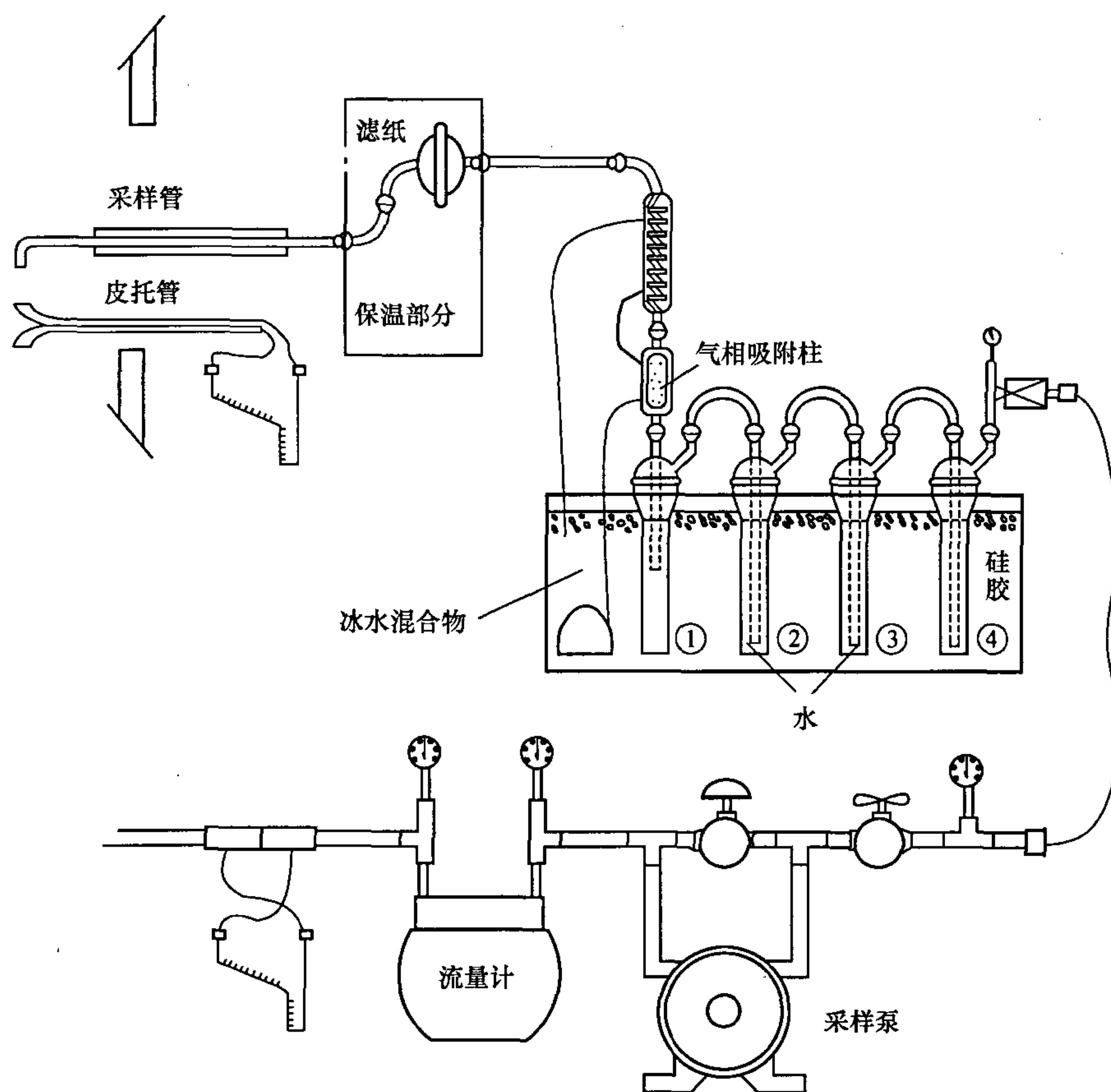
图 B.3 废气采样装置 II
