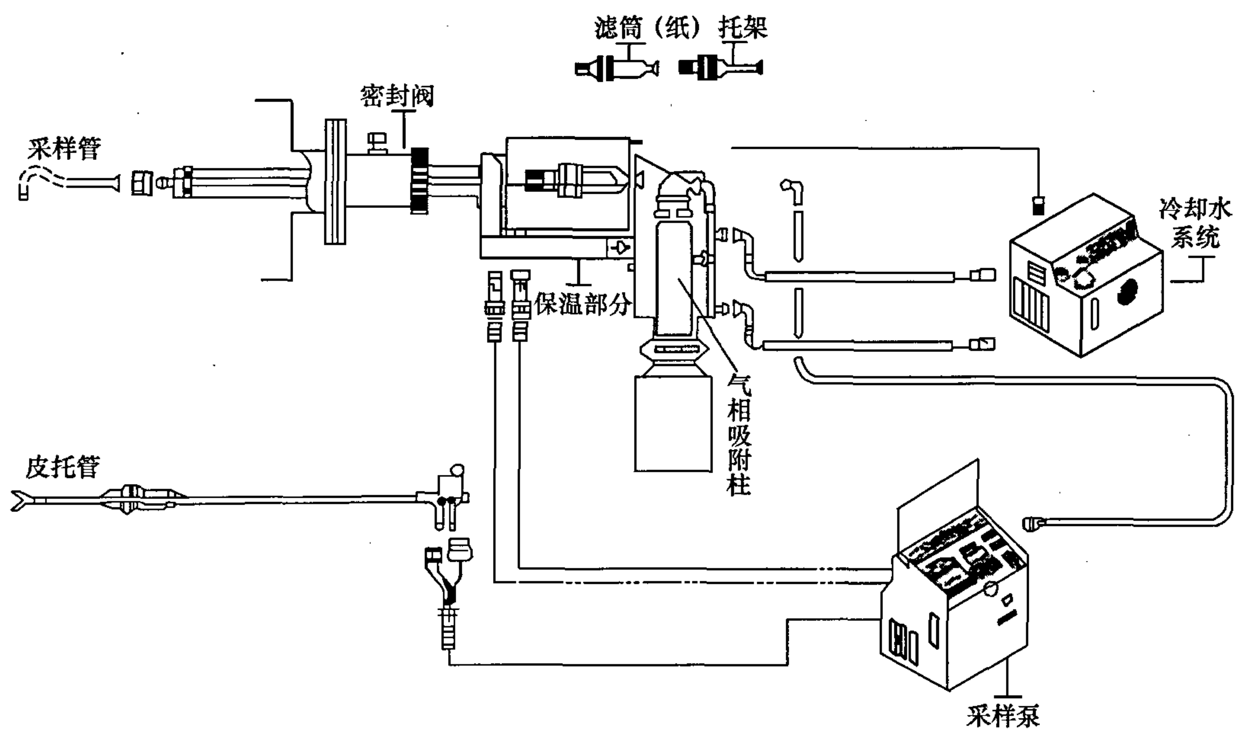
图 B.4 废气采样装置 III
