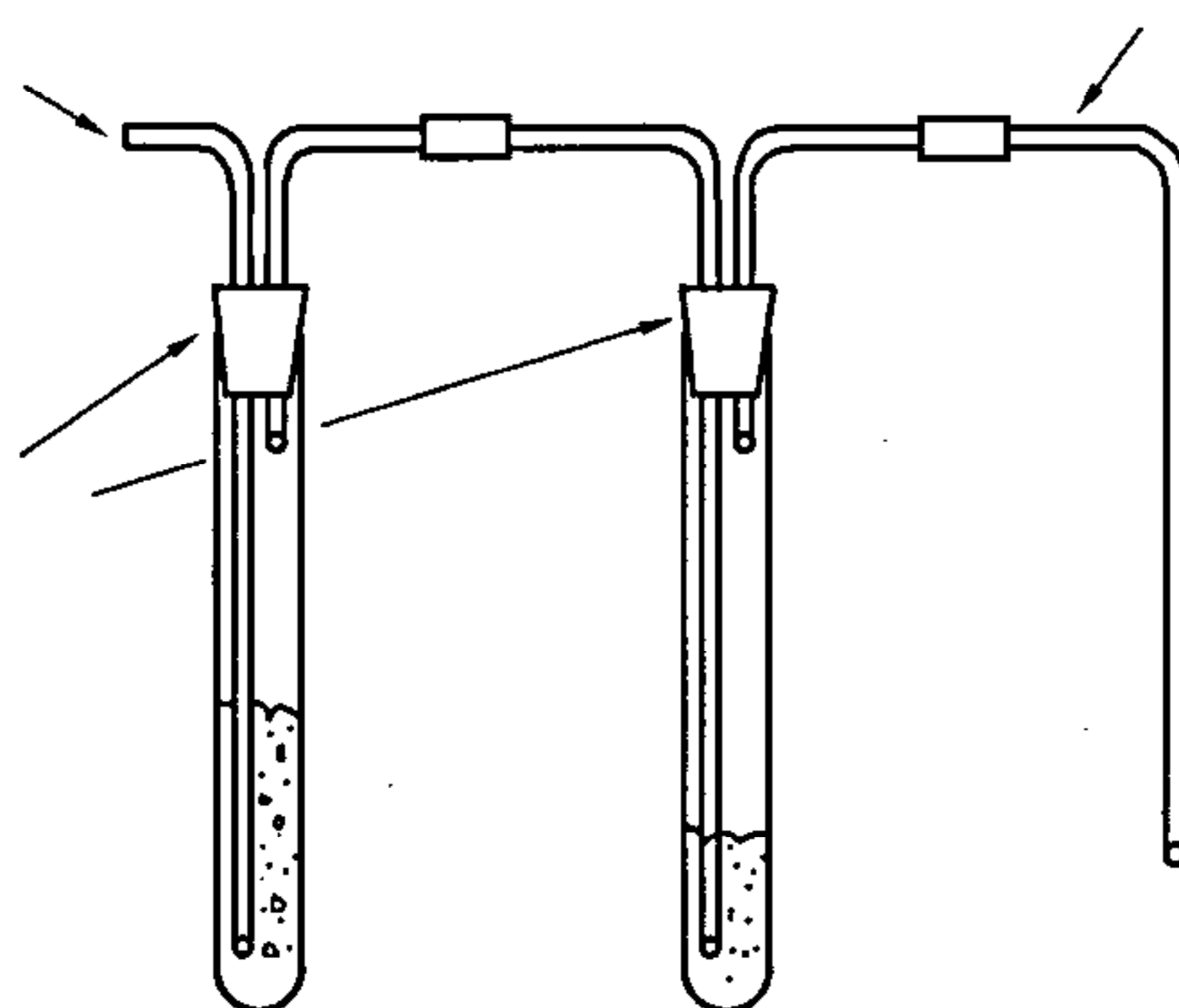
图 N.1 重氮甲烷发生装置
